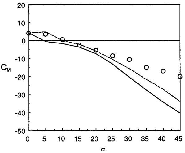
(D) M = 2.87, \delta_w = 20^\circ, \phi = 0^\circ
