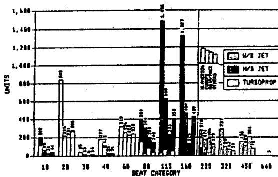
Figure 1.1 Actual Fleet—1987
