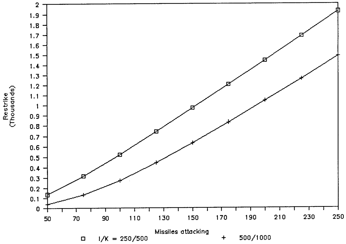
Fig. 23 Restriking RVs
