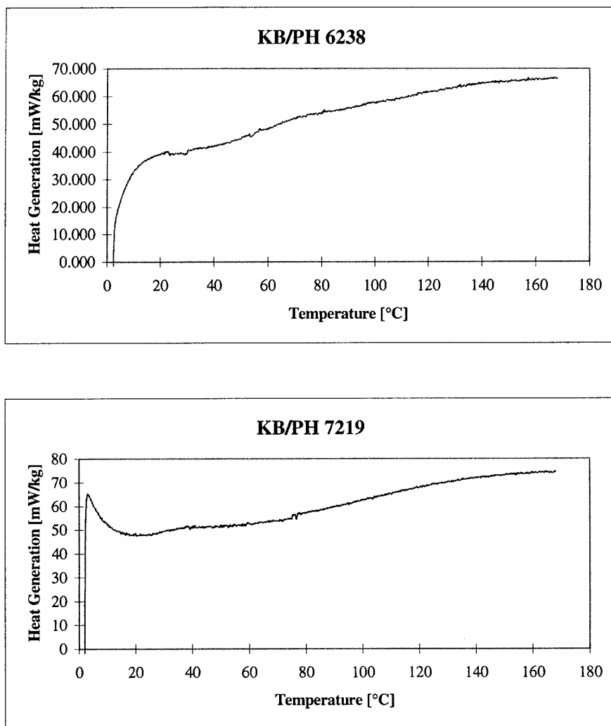
Figuur A.1: Warmteontwikkelingscurve van KB/PH 6238 en KB/PH 7219.
