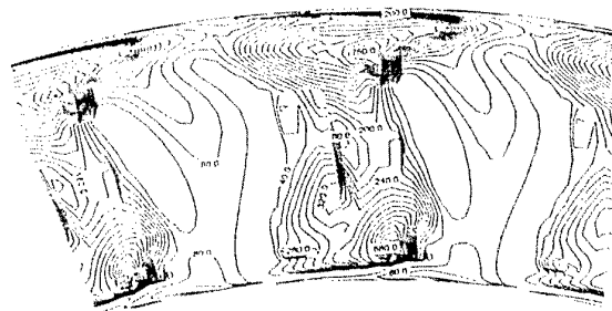
(d) CANARI using k-\epsilon turbulence model (Couaillier)
