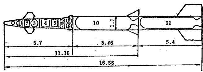
图5-7 “斯巴坦”的外形与结构示意图 1—战斗部；2—舵机；3—发动机；4—能源；5—电源；6—控制系统； 7—自动驾驶仪；8—稳定平台；9—计算机； 10—主发动机；11—加速器。
