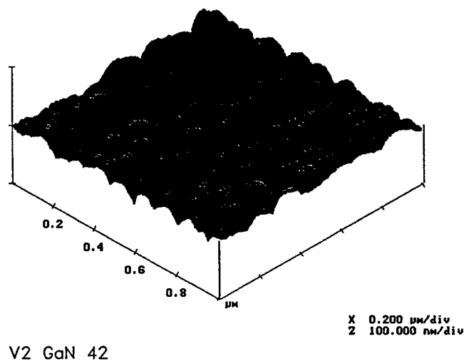
Fig. 9 AFM
