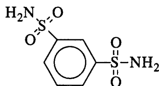
1,3-benzenedisulfonamide (BDSA)
