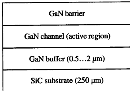
Fig. 1: MODFET epi structure
