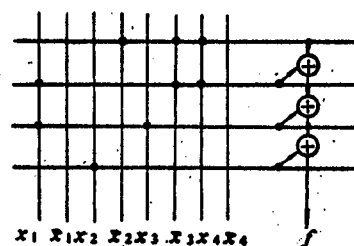
Fig. 7 R-PLA circuit of f(x_1, x_2, x_3, x_4)
