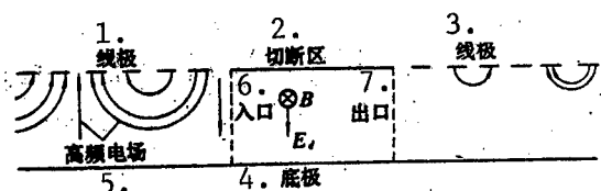
图2 切断区示意图
