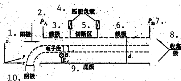
图1 IBCFA 器件结构示意图
