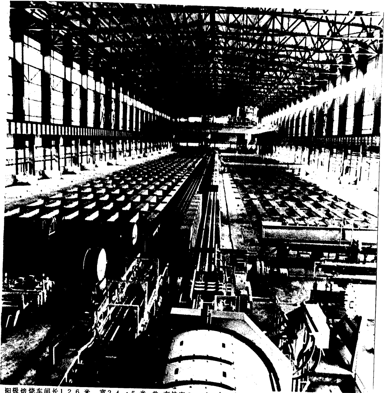
阳极焙烧车间长126米，宽24.5米，共有炉室68个，在工人们精心操作下，生产情况良好。
