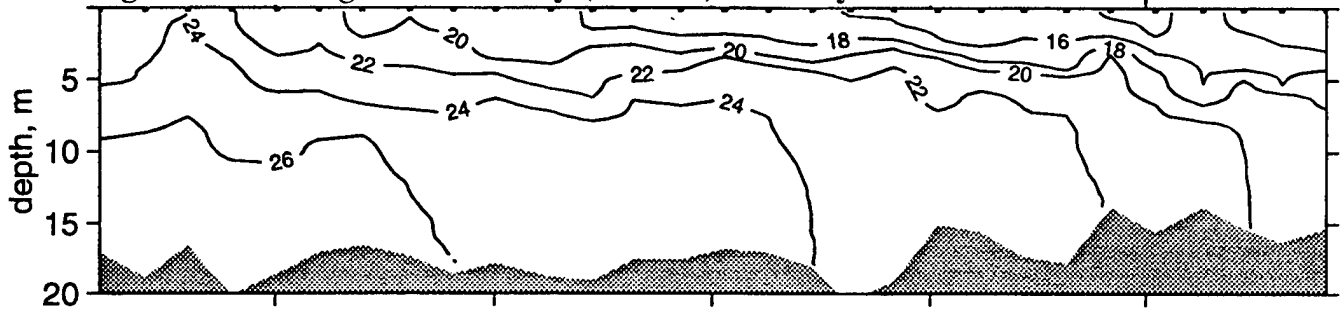
Figure 39a. Longitudinal Survey (10/20/95): Salinity Contour
