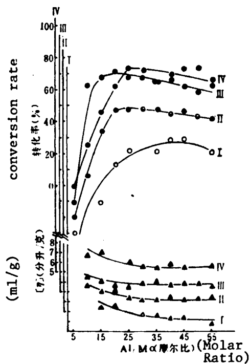
I. \text{MoCl}_4(t\text{-OC}_2\text{H}_5)_{4-n} ; II. \text{MoCl}_4(\text{S-OC}_2\text{H}_5)_{4-n} ; III. \text{MoCl}_4(i\text{-OC}_2\text{H}_5)_{4-n} ; IV. \text{MoCl}_4(i\text{-OC}_3\text{H}_7)_{4-n}
