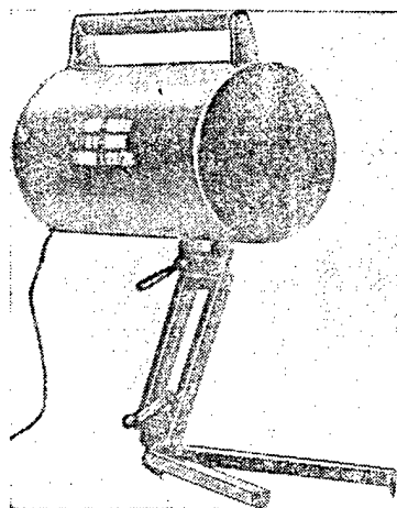
Рис. 3. Австрийская противобортовая мина SMI 22/6
