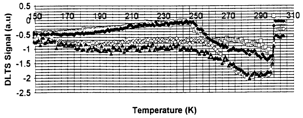
Fig. 17 DLTS scan for trap T E2
