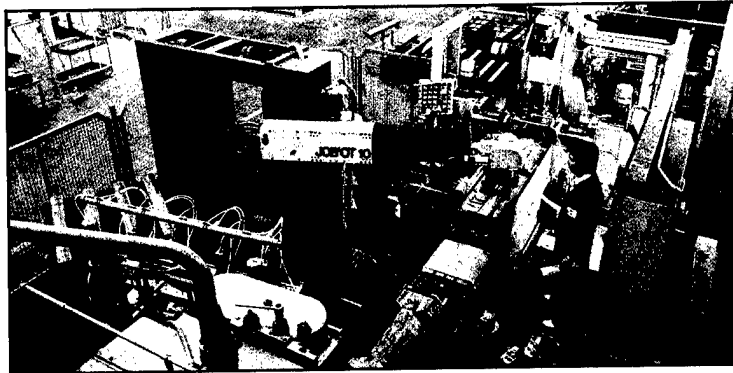
Robot de manutention et d'égavurage pour pièces de carrosserie. 8 axes et une tête de fraisage en option. (Doc. Jobs)
