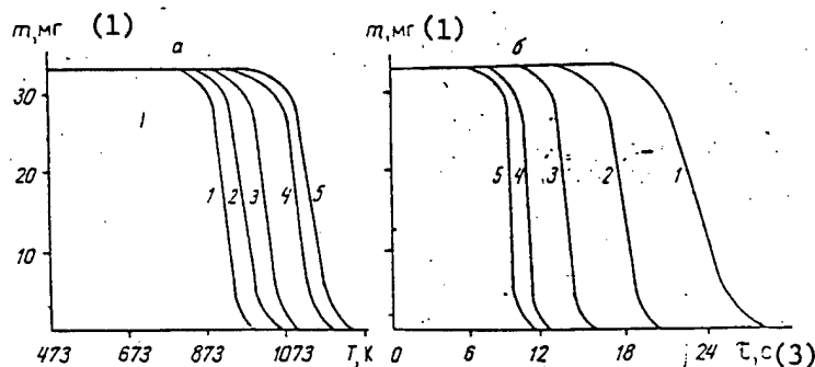
Рис. 2. Зависимость потерь массы образцов политрифторхлорэтилена от температуры в термокамере (а) и времени (б): 1—923 К, 2—1073, 3—1098, 4—1148, 5—1273 К
