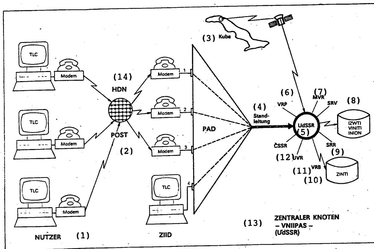
1 Struktur des Datenbank- und Datenkom- munikationsnetzes der RGW-Länder
