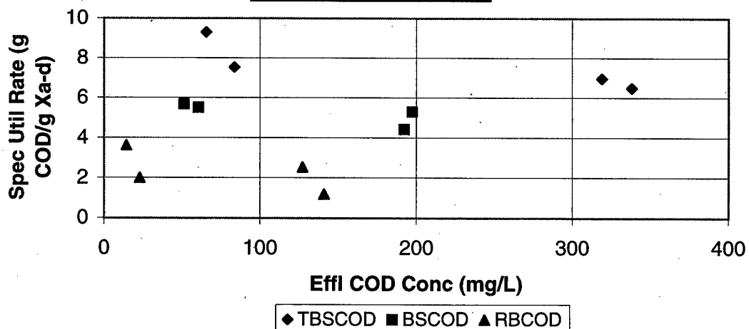
Effl COD Conc vs SUR
