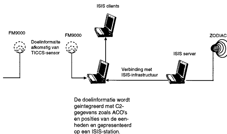
Figuur 17: Doelinformatie gecombineerd met C2-gegevens weergegeven op een ISIS-station.
