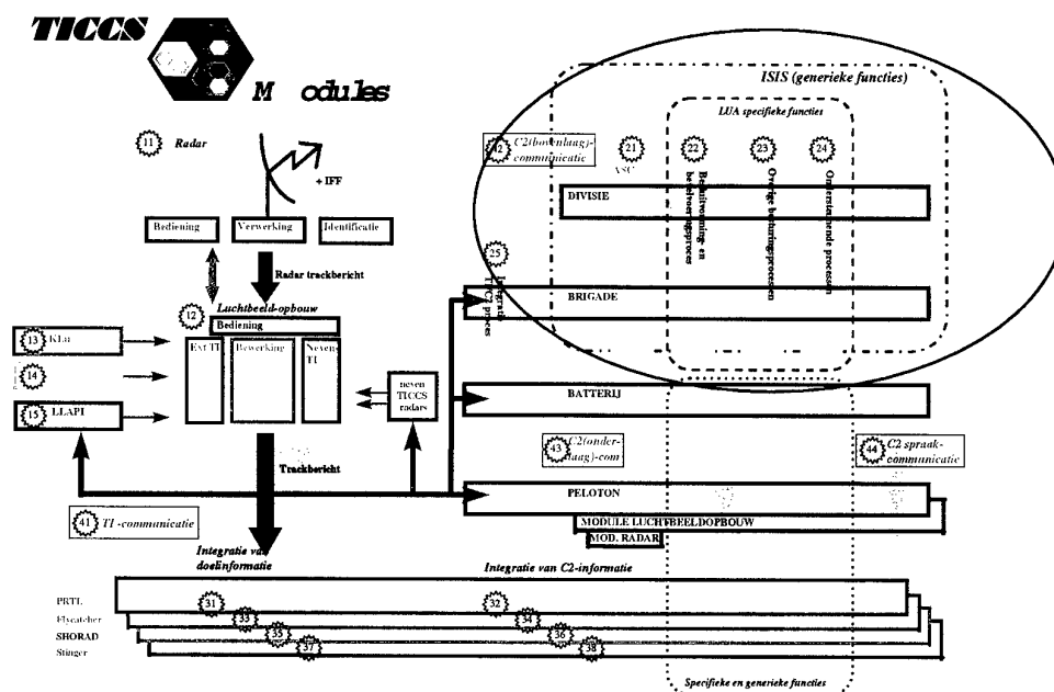
Figuur 8: De TICCS componenten met omcirkeld de C2-bovenlaag.
