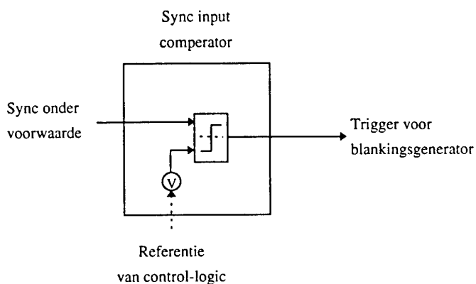
Figuur 3.3: Sync input comperator
