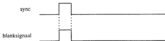
Figuur 2.11: Mode 1: Extern bepaalde blankingstijd
