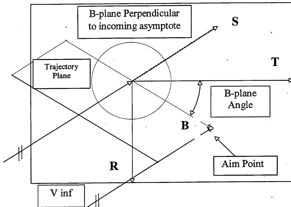
Figure 2.3: Mars B-Plane
