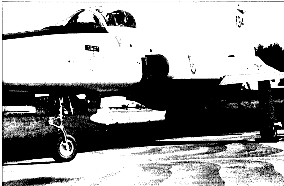
Fig. 2: The programmable EW pod
