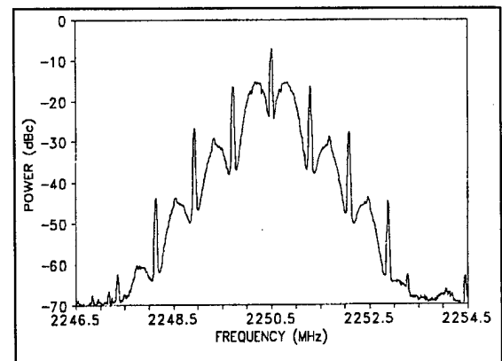
Figure A-4. Bi \phi PCM/PM signal.
