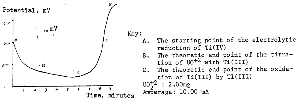
Fig. 3 Ti(III) - Tl(III) Biintermediate Coulometric Titration of Uranium
