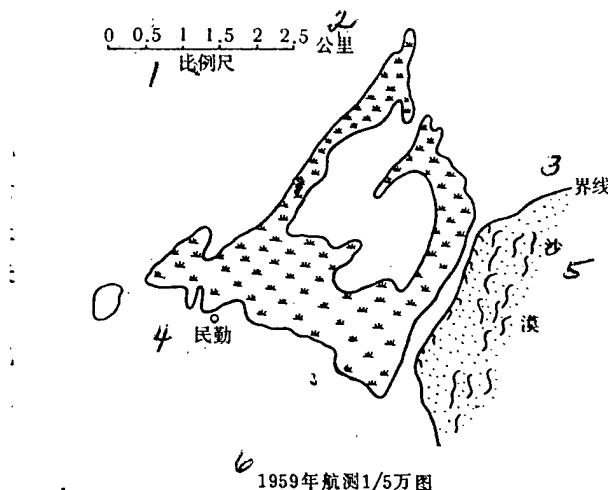
图7 民勤绿洲与沙漠的间距示意图
