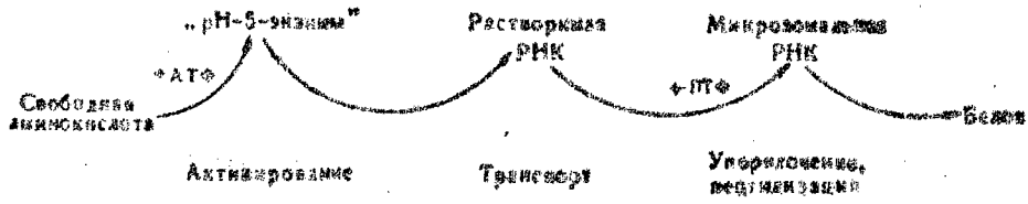
Рис. 3. Этапы синтеза белка
