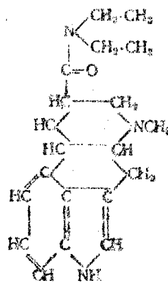
Диэтил-амид лизерговой кислоты
