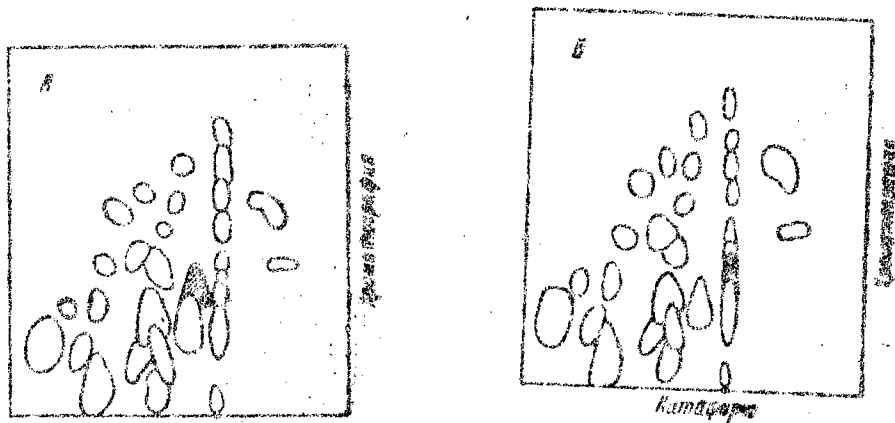
Рис. 6. «Химическая дактилоскопия» гемоглобинов. А — серповидный гемоглобин, В — нормальный гемоглобин
