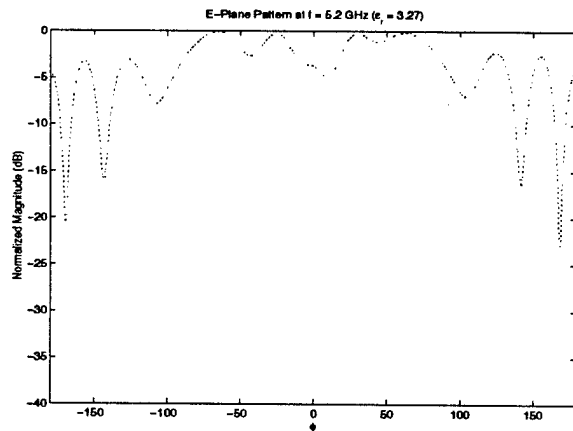
(d) E-Plane pattern at f = 5.2 \text{ GHz}
