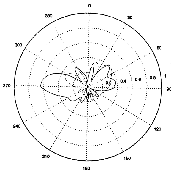
(d) d=0.8\lambda_d , w=0.85\lambda_d
