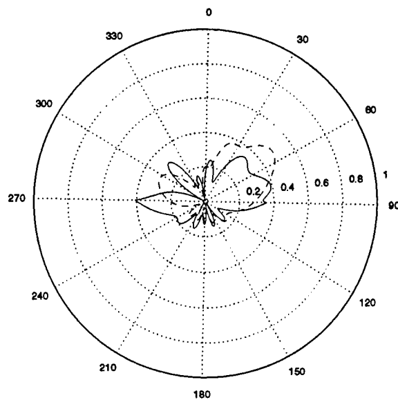
(b) d=0.6\lambda_d , w=0.85\lambda_d
