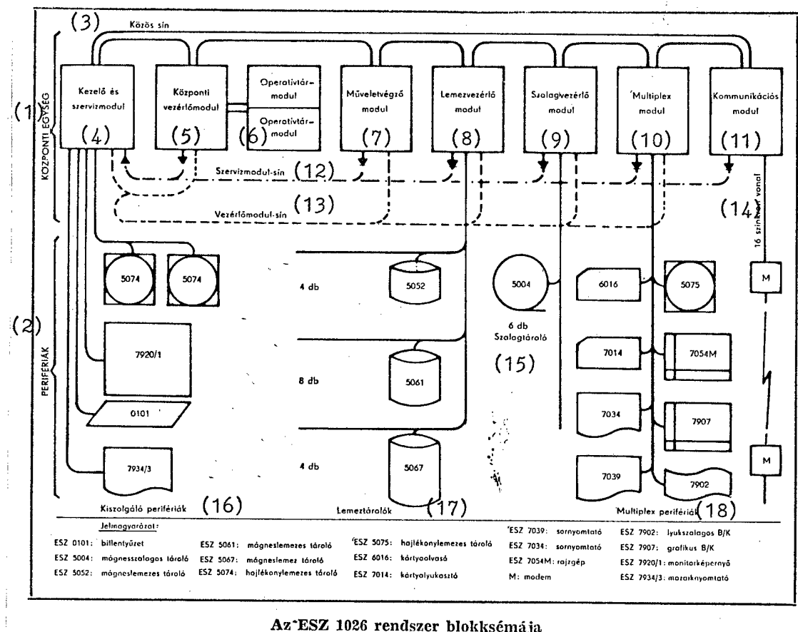
Az ESZ 1026 rendszer bloksémája
