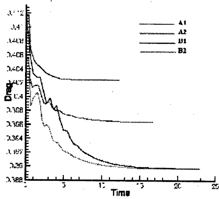
Fig. 17. Q=2.4 kW.
