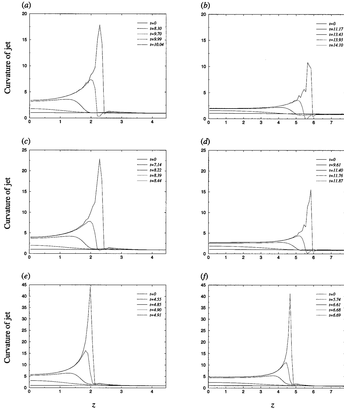
Figure 10: Variation of the curvature of the jet, Re=200 , \varepsilon_o=0.5 , s=10^{-3} : (a) k=0.7 , \beta=0 ; (b) k=0.4 , \beta=0 ; (c) k=0.7 , \beta=1 \times 10^{-2} ; (d) k=0.4 , \beta=1 \times 10^{-2} ; (e) k=0.7 , \beta=3 \times 10^{-2} ; (f) k=0.4 , \beta=3 \times 10^{-2} .
