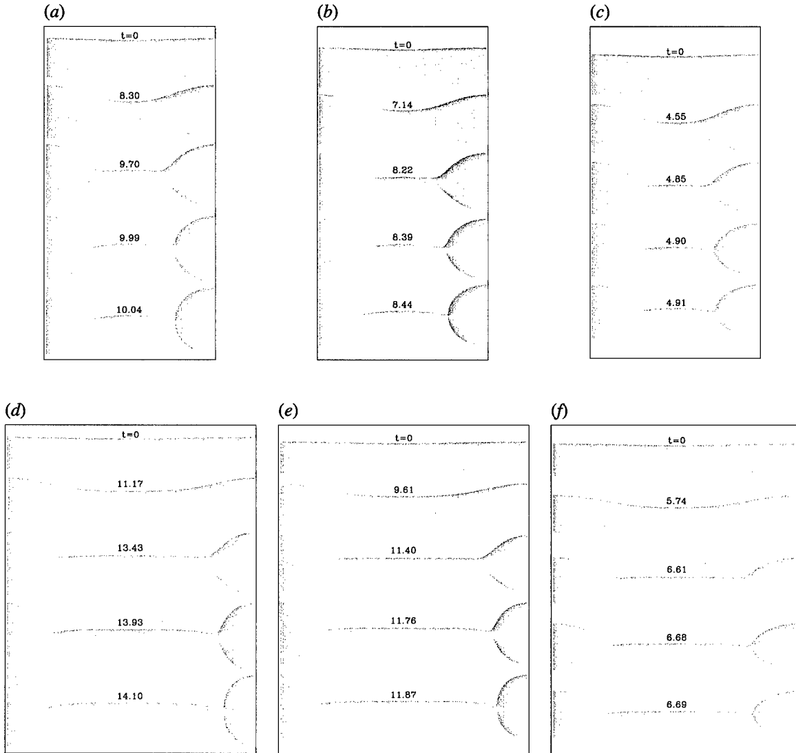
Figure 2: Time evolution of the instability, Re=200 , \varepsilon_0=0.5 , s=10^{-3} : (a) k=0.7 , \beta=0 ; (b) k=0.7 , \beta=10^{-2} ; (c) k=0.7 , \beta=3 \times 10^{-2} ; (d) k=0.4 , \beta=0 ; (e) k=0.4 , \beta=10^{-2} ; (f) k=0.4 , \beta=3 \times 10^{-2} .
