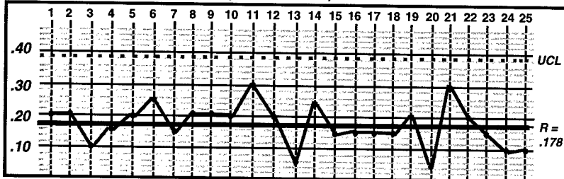
R (Control Chart)*
