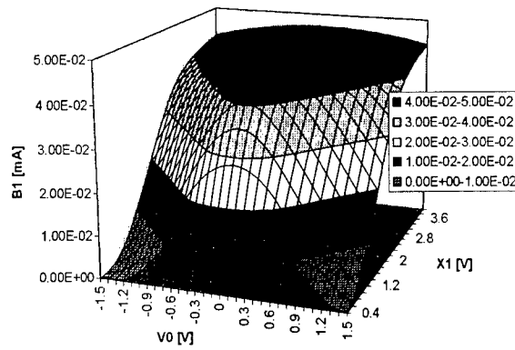
Fig. 5.a , Fundamental magnitude
