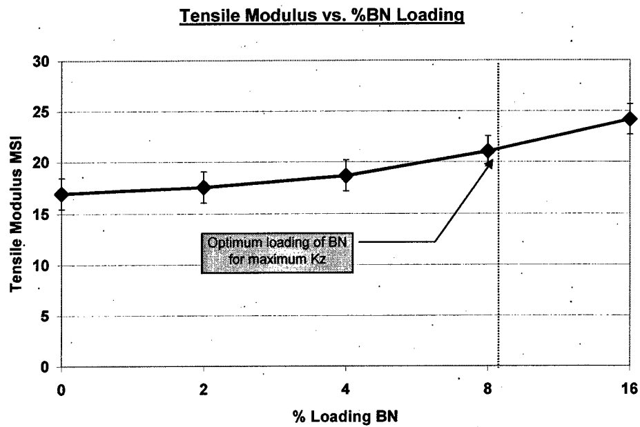
Figure 7. Tensile modulus
