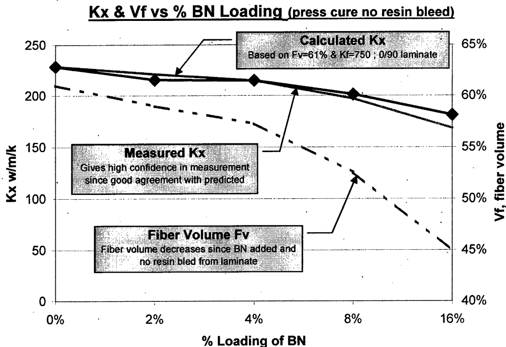
Figure 5. Kx & Vf vs % BN loading
