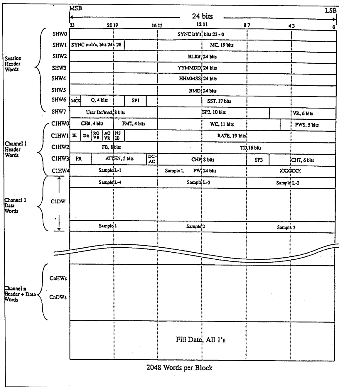
Figure 6-8. ADARIO data format.
