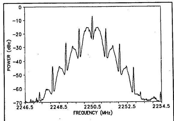
Figure A-4. Bi \phi PCM/PM signal.
