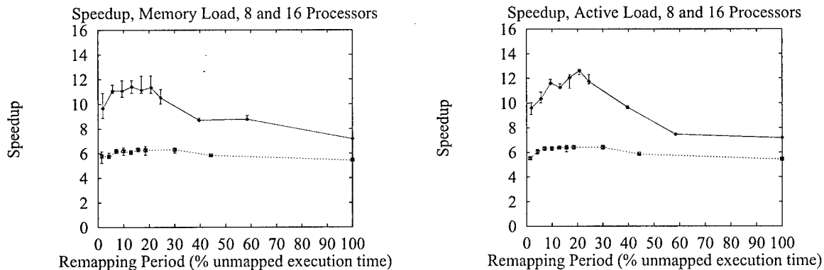
FIG. 6.3. Speedups
