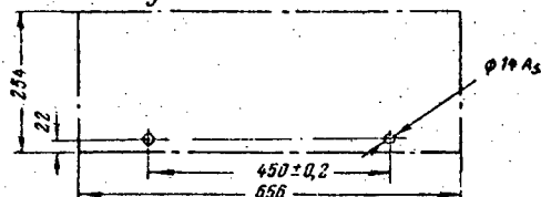
Разметка для крепления стойки к полу
