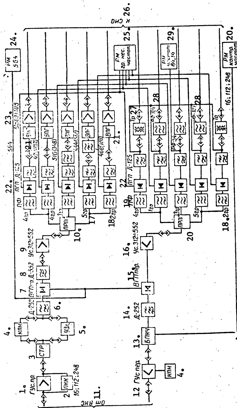
Рис. IV.7.3. Блок-схема стойки групповых устройств СГУ аппаратуры К-60
