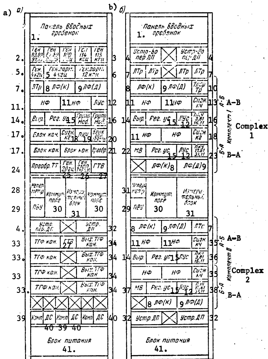
Рис III.5.3. Размещение оборудования на стойке оконечной (а) и промежуточной (б) станций аппаратуры БО-3-2
