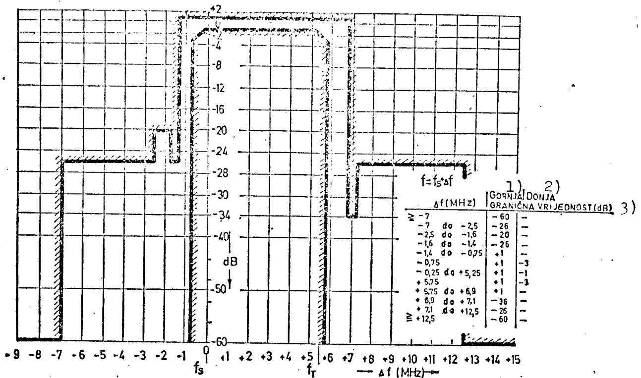
4.) Opseg frekvencije I i III
