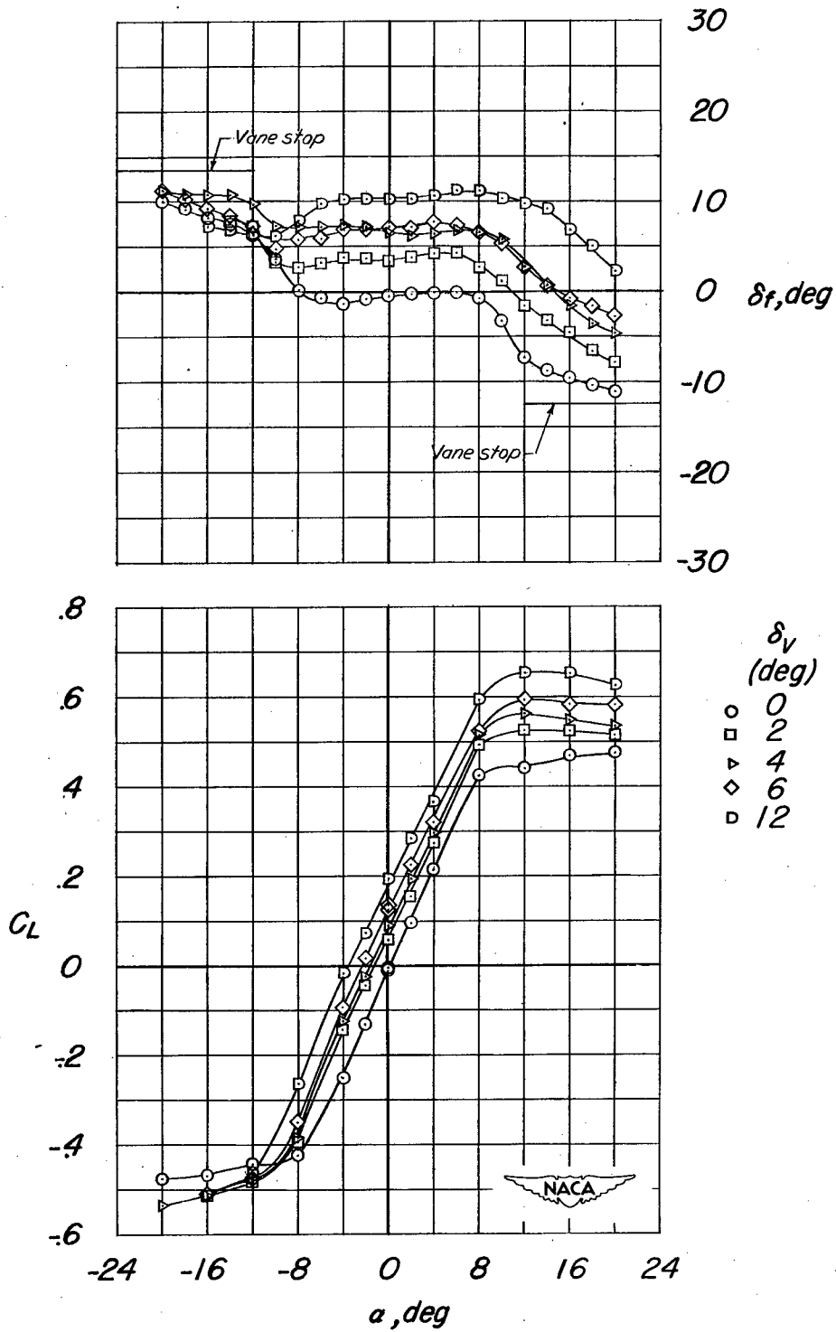
(d) M = 0.90 .
