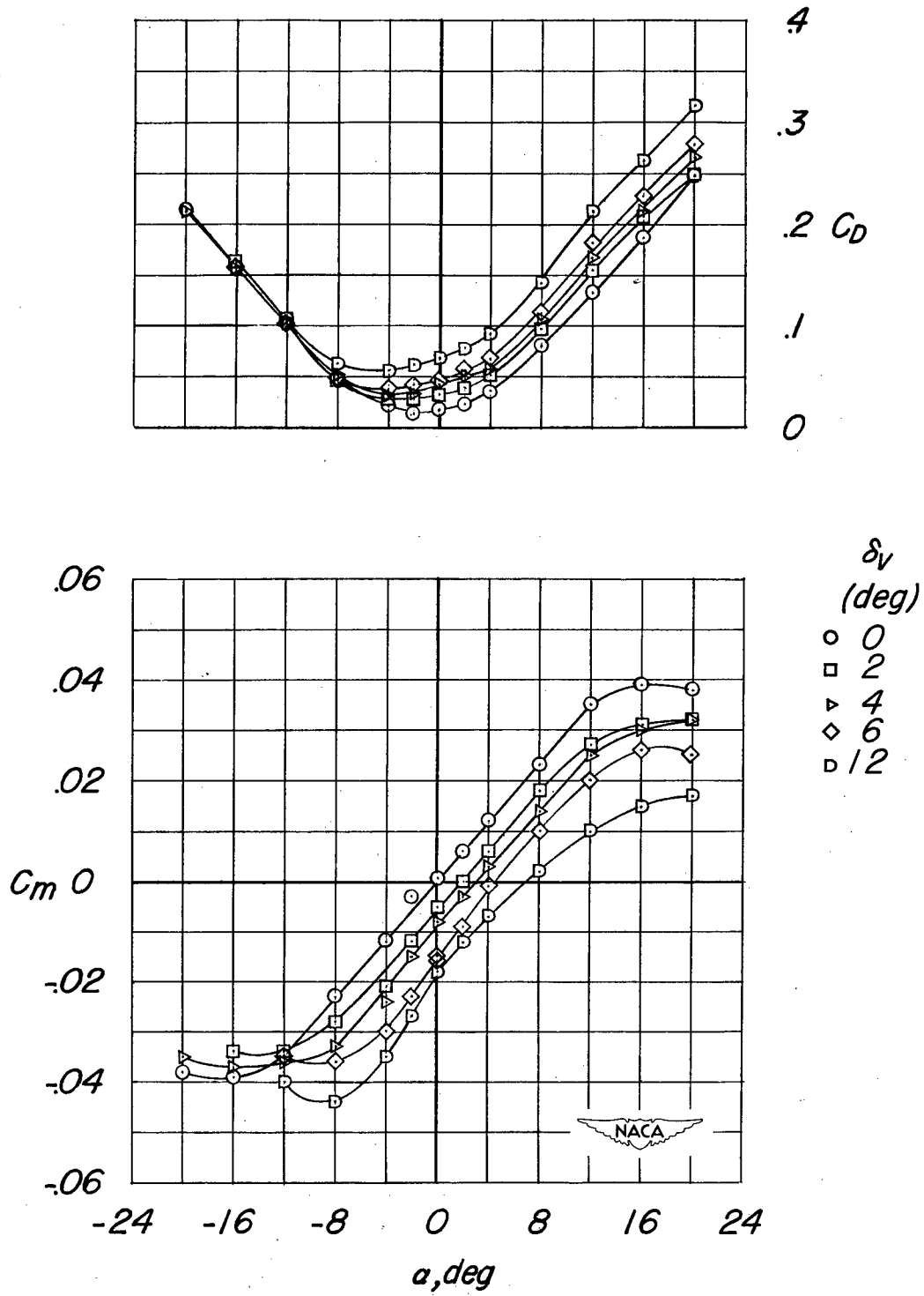
(d) M = 0.90 .
