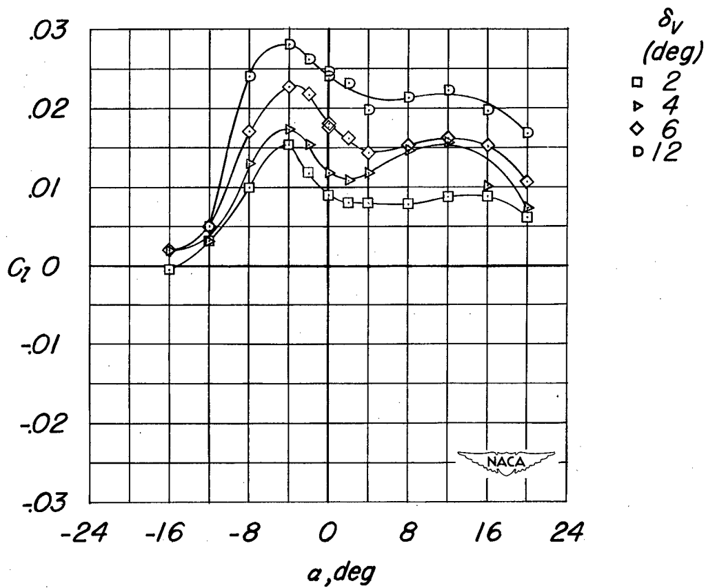
(d) M = 0.90 .
