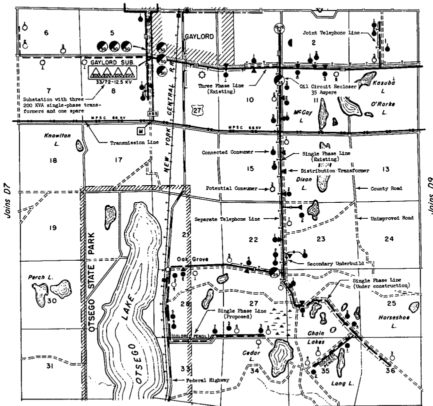
FIGURE VI. Detail map.
