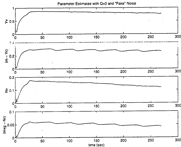
Figure 4-7: Parameter Estimates
