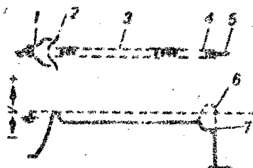
Fig. 8. Setup of the Hines experiment: 1) cathode; 2) anode; 3) axial coil; 4) electron collector; 5) ion collector; 6) ionic trap; 7) ion extraction.
