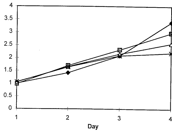
B: scFv-Fc
