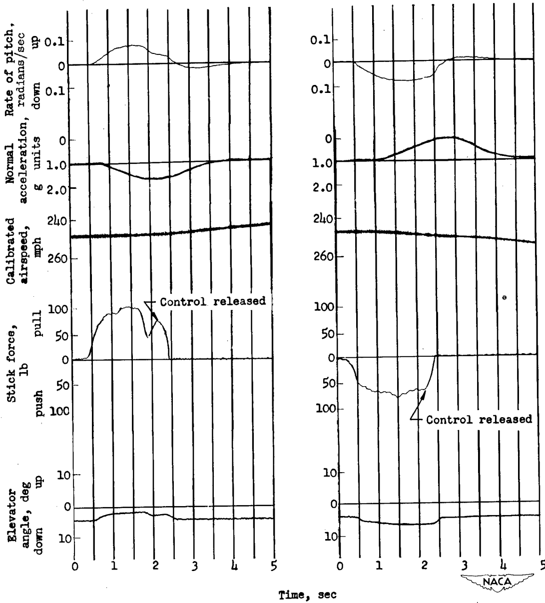
(d) Feel-device setting C.
