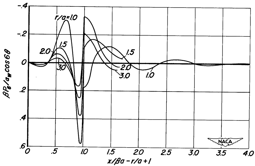
(d) n = 3
