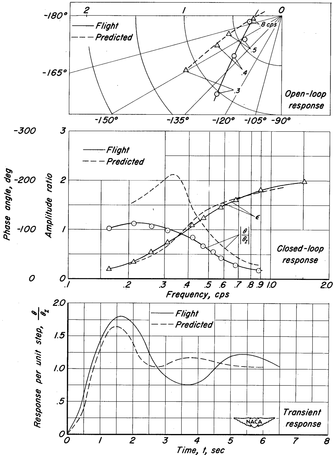
(d) 130 knots, sensitivity 63 percent, rate 0.
