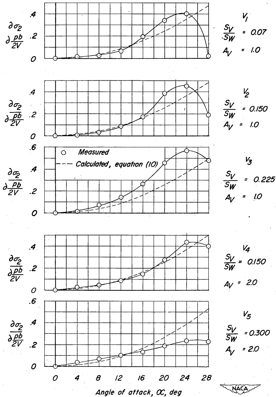
(a) Fuselage F_2 .
