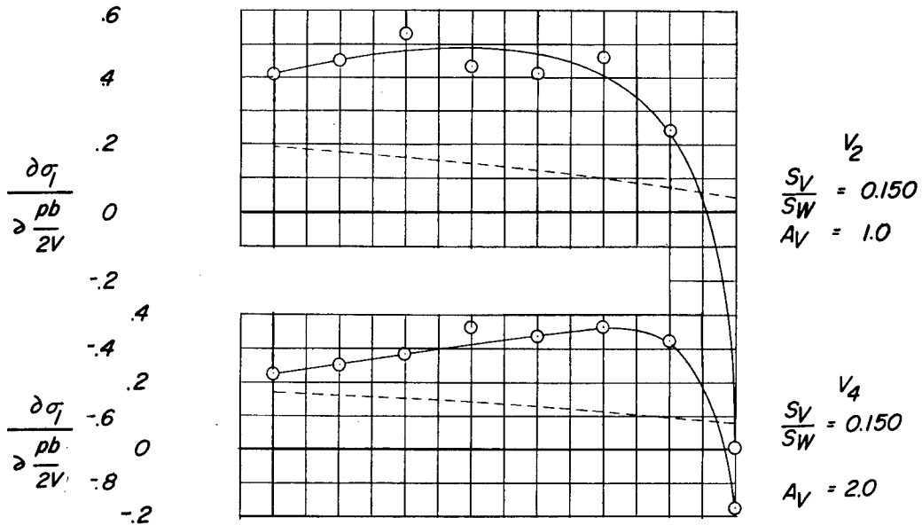
(b) Fuselage F 1 .
