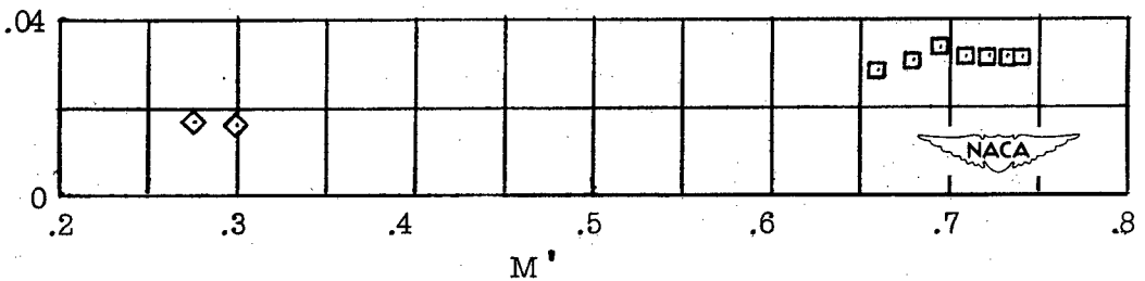
(d) Lift coefficient from 0.30 to 0.40.
