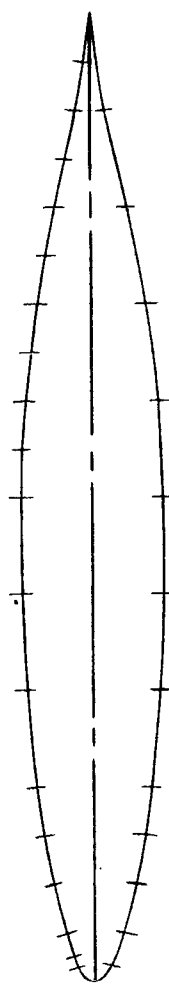
NACA 66,2-015
